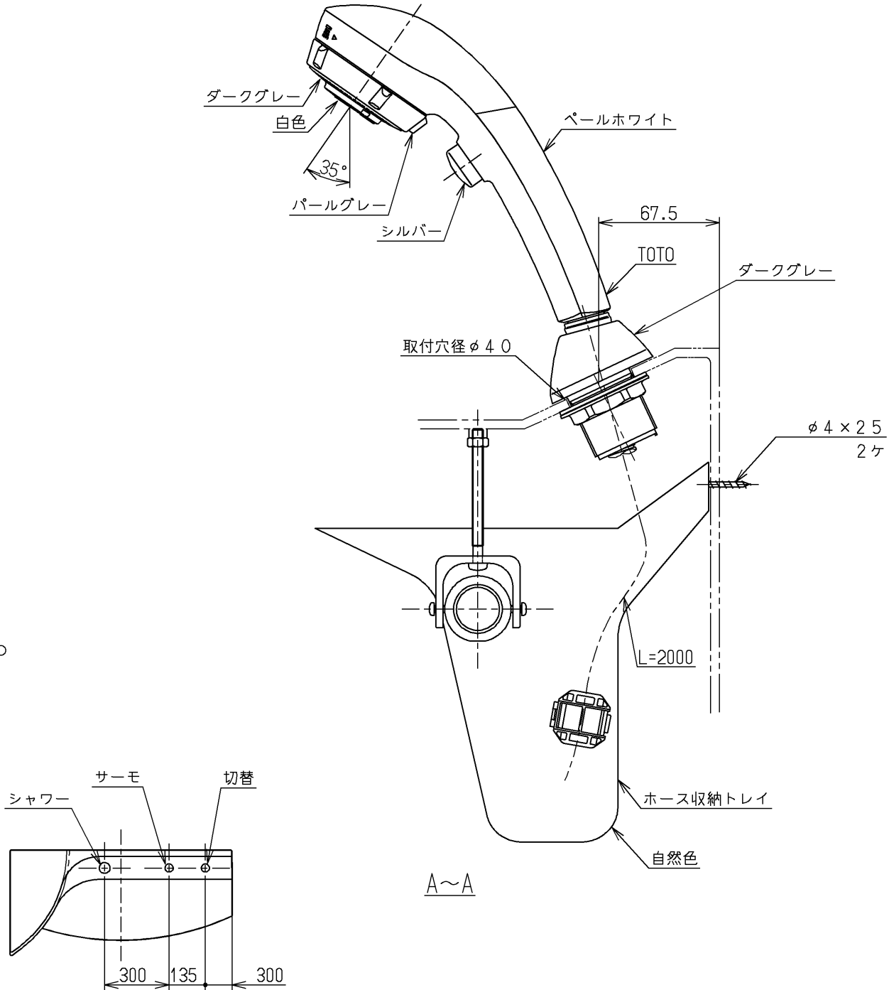
水栓取付け位置（フリー）
